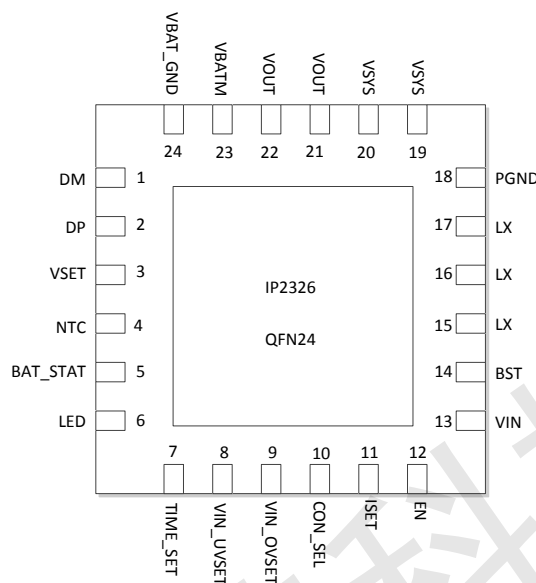
图 2 IP2326 引脚图
